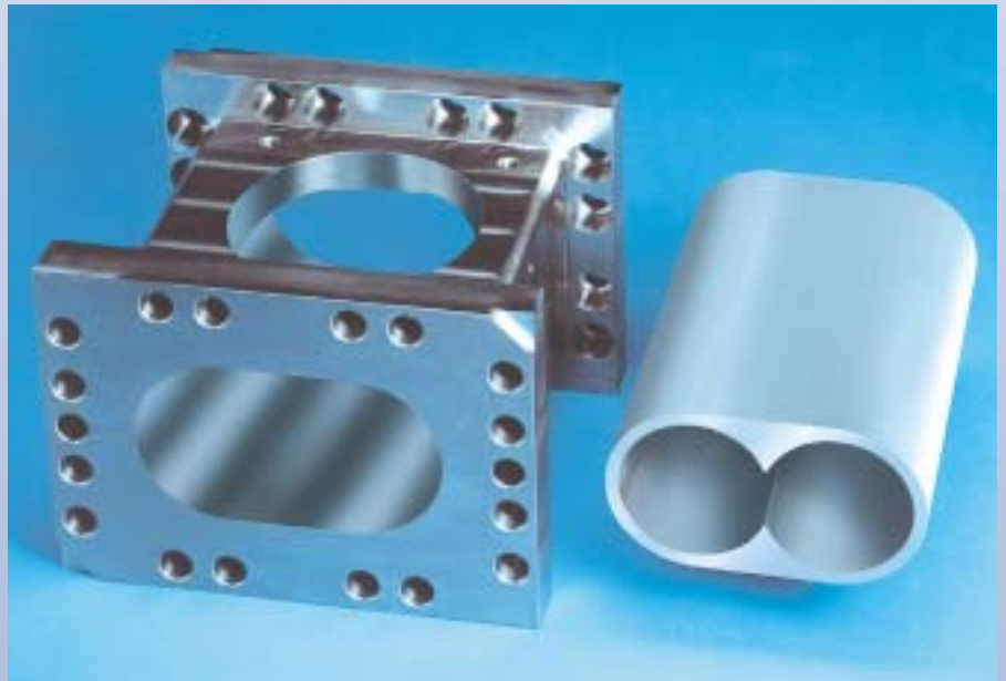
Doppelschneckengehäuse mit Verschleißeinsetzung
